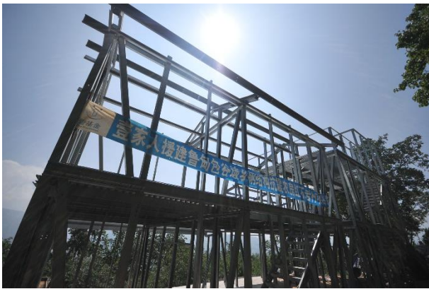
图为巧家县包谷垭乡钢结构抗震农房红石岩村项目点
